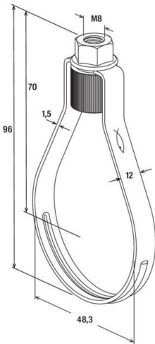
Maßzeichnung
