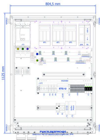
Maßzeichnung
