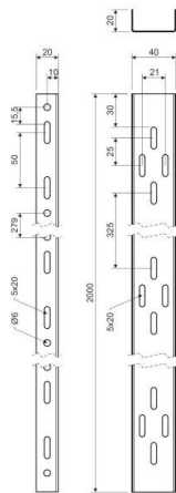
Maßzeichnung
