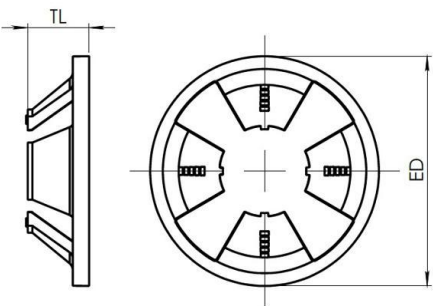
Maßzeichnung
