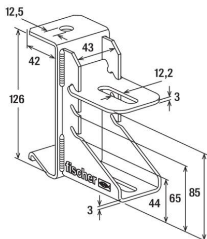
Maßzeichnung
