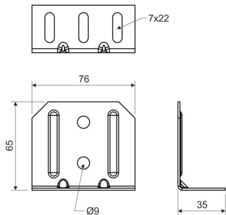
Maßzeichnung
