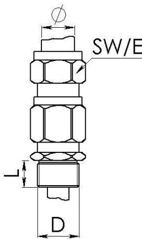
Maßzeichnung
