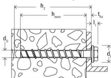
Strichzeichnung
