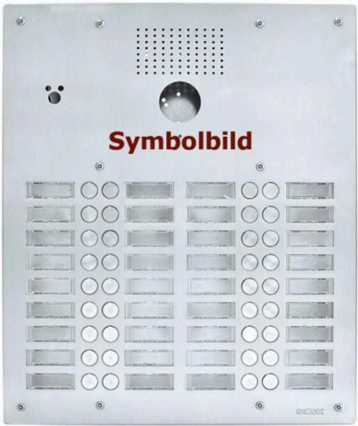
Türstation UP silber Antivandal VIDEO 4-reihig mit 28 Tasten und Bohrung P1, FERMAX
