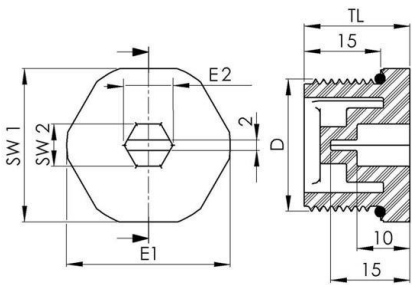
Maßzeichnung
