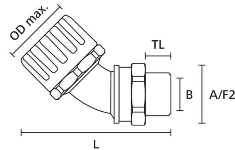
Maßzeichnung
