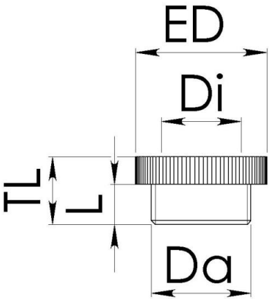
Maßzeichnung
