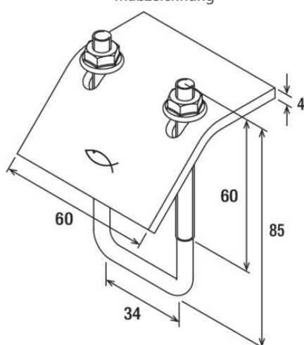
Maßzeichnung
