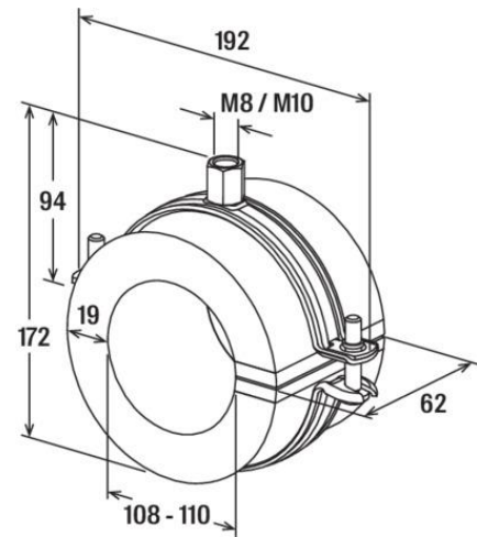
Maßzeichnung
