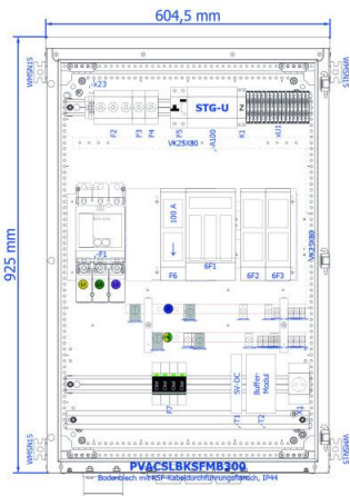
Maßzeichnung
