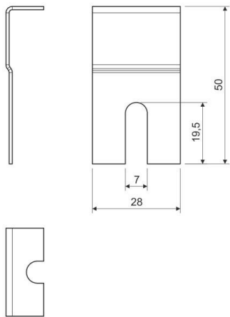
Maßzeichnung
