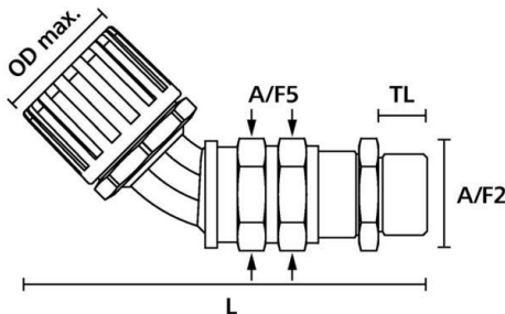
Maßzeichnung
