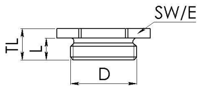
Maßzeichnung
