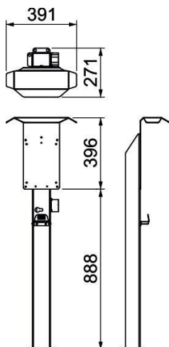
Maßzeichnung
