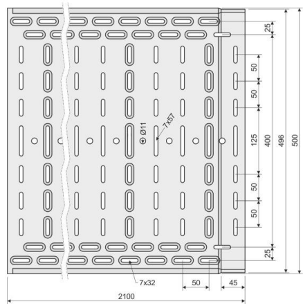
Maßzeichnung
