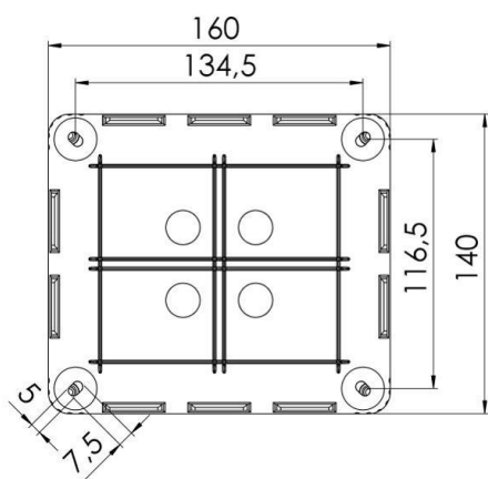
Maßzeichnung
