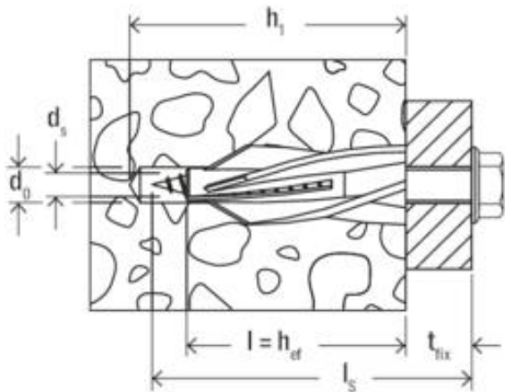
Strichzeichnung
