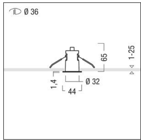
Maßzeichnung
