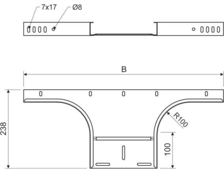
Maßzeichnung
