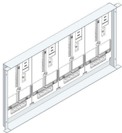
Zählerwanne mit Zählerplatte
