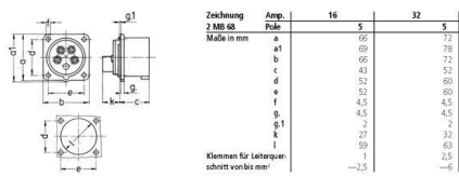
Maßzeichnung
