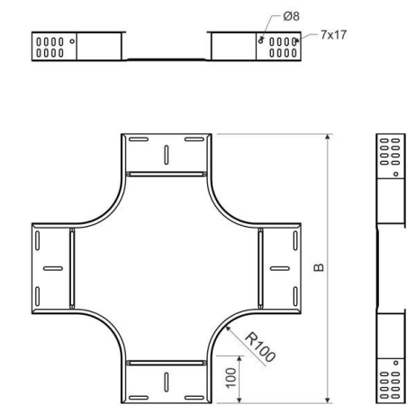
Maßzeichnung
