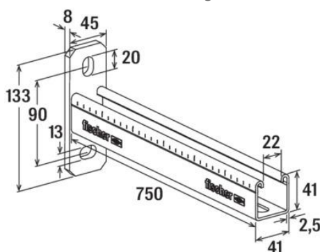
Maßzeichnung
