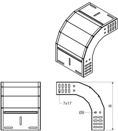
Maßzeichnung
