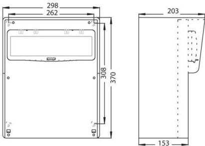
Maßzeichnung
