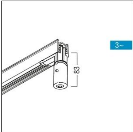
Maßzeichnung
