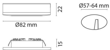
Maßzeichnung
