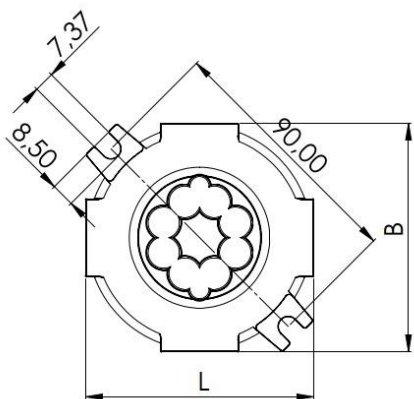
Maßzeichnung
