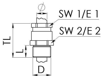
Maßzeichnung
