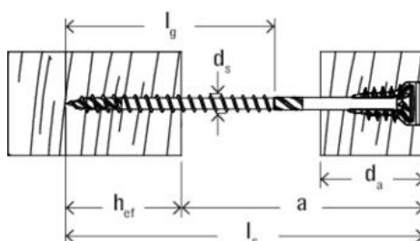
Strichzeichnung
