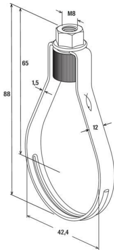
Maßzeichnung
