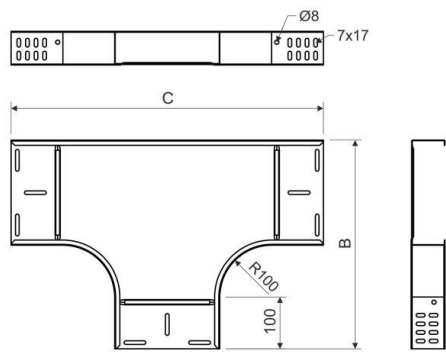
Maßzeichnung
