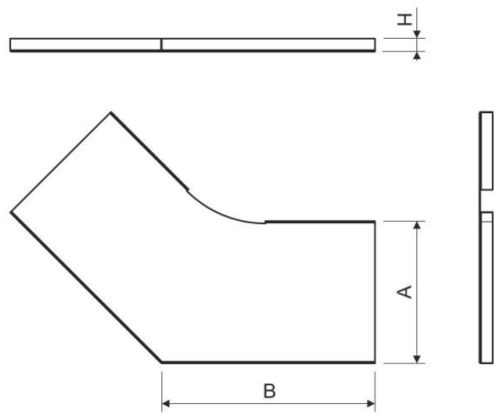
Maßzeichnung
