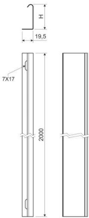
Maßzeichnung
