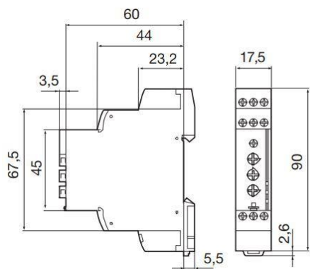
Maßzeichnung
