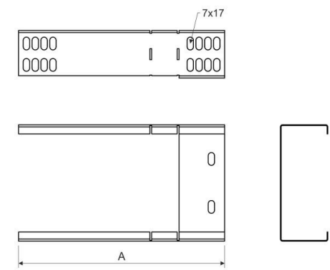
Maßzeichnung
