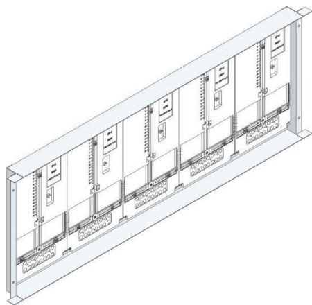
Zählerwanne mit Zählerplatte
