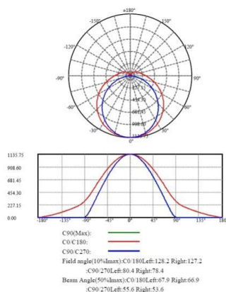
Lichtverteilungskurve
