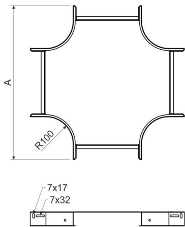
Maßzeichnung
