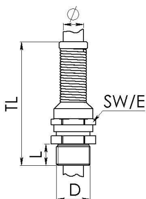
Maßzeichnung
