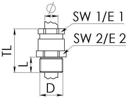
Maßzeichnung
