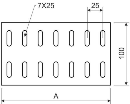
Maßzeichnung
