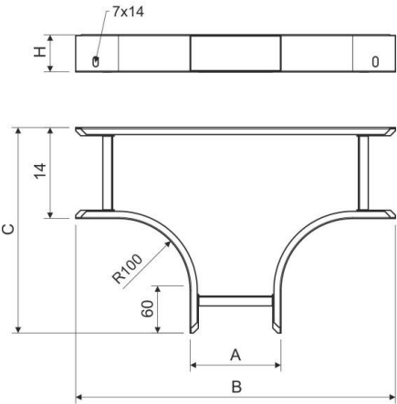
Maßzeichnung
