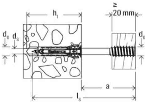
Strichzeichnung
