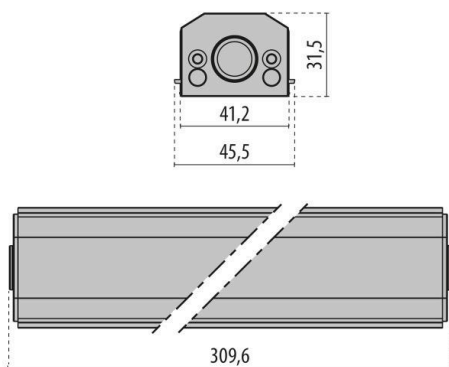
Maßzeichnung
